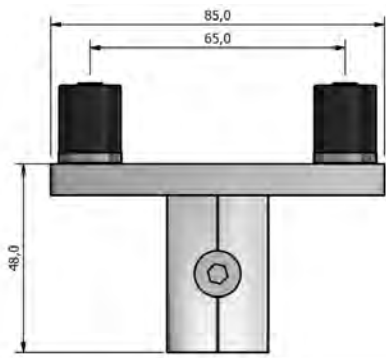
Vistafold® Mullion Guide
